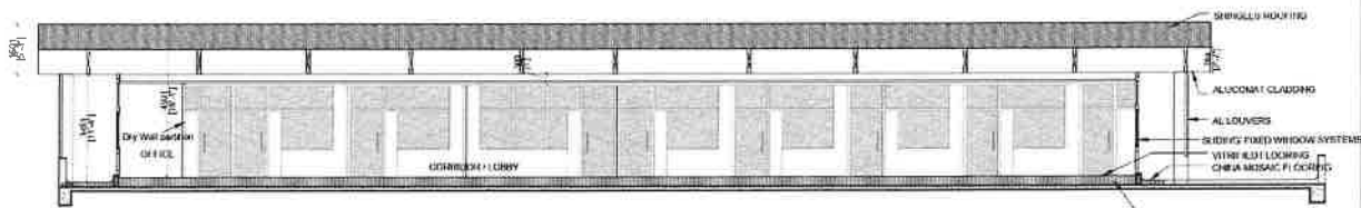
SECTION A-A'
